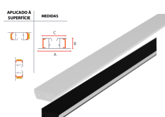
STYLUS 75x25 SOBRREPOR - 2000mm
