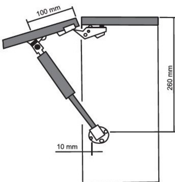
Porta à 75°
