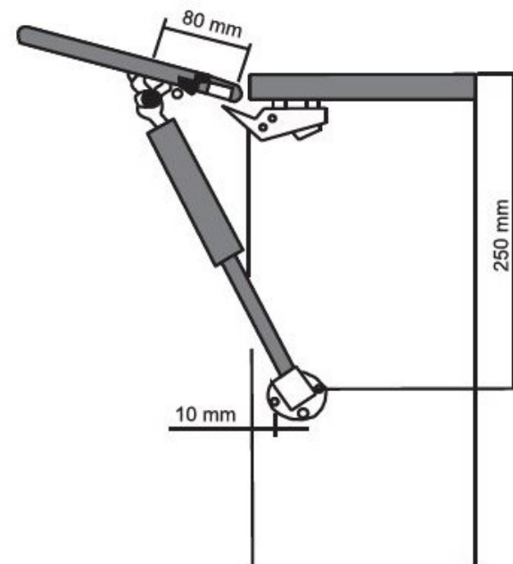
Porta à 110°
